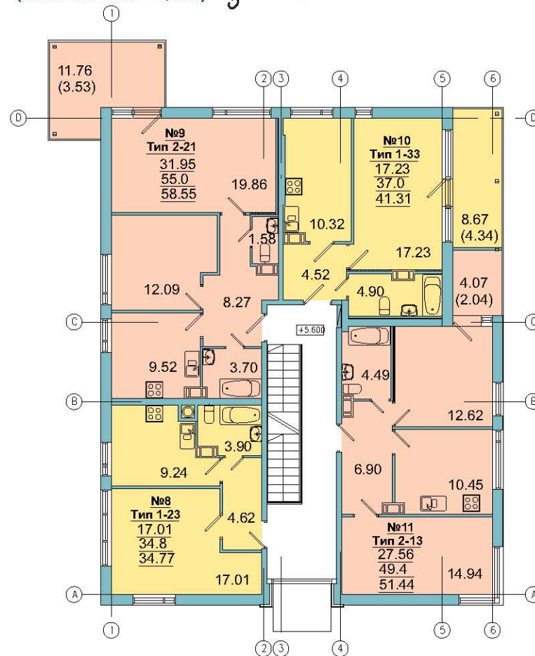
3 этаж (План на отм. +5,600)
