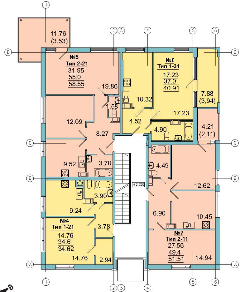
2 этаж (План на отм. +2,800)
