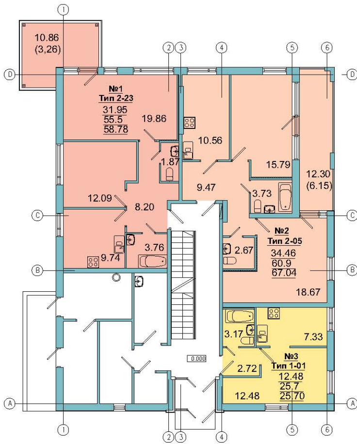
1 этаж (План на отм. 0,000)
