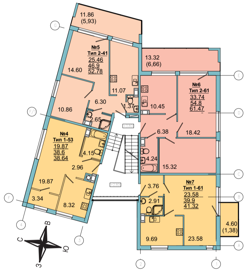
3 этаж (План на отм. +5,600 и +6,600)
