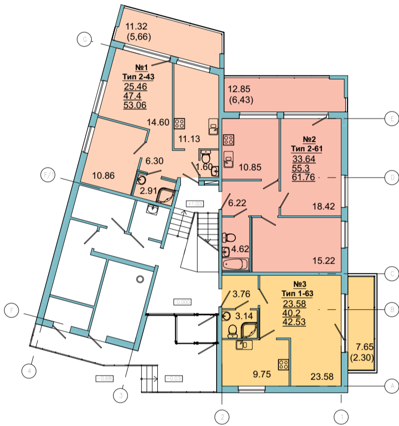
1 этаж (План на отм. 0,000 и +1,000)
