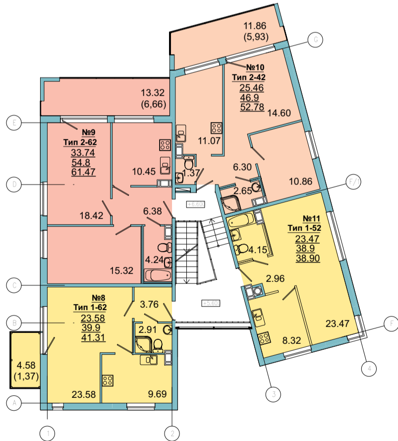
3 этаж (План на отм. +5,600 и +6,600)
