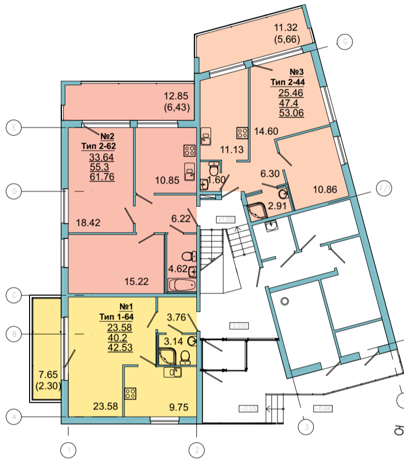
3 этаж (План на отм. +5,600 и +6,600)
