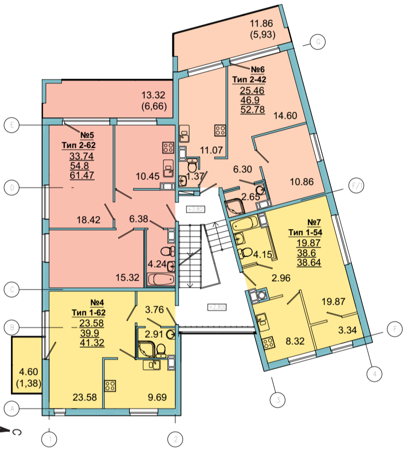
2 этаж (План на отм. +2,800 и +3,800)
