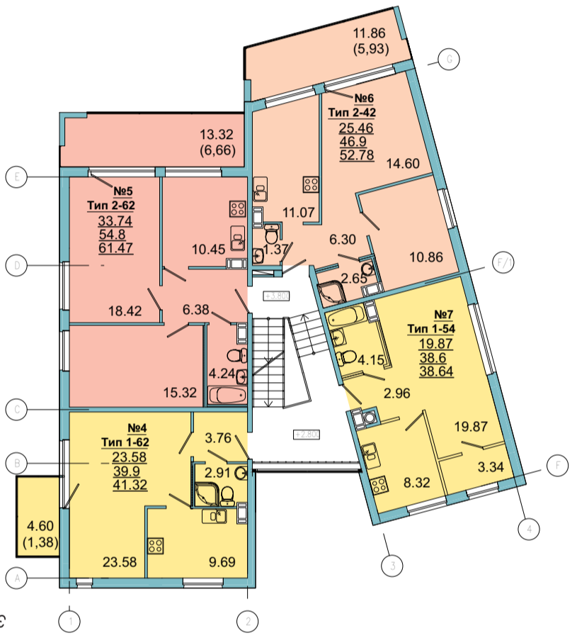
2 этаж (План на отм. +2,800 и +3,800)
