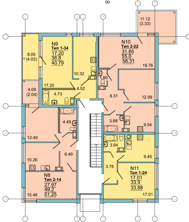
3 этаж (План на отм. +5,600)
