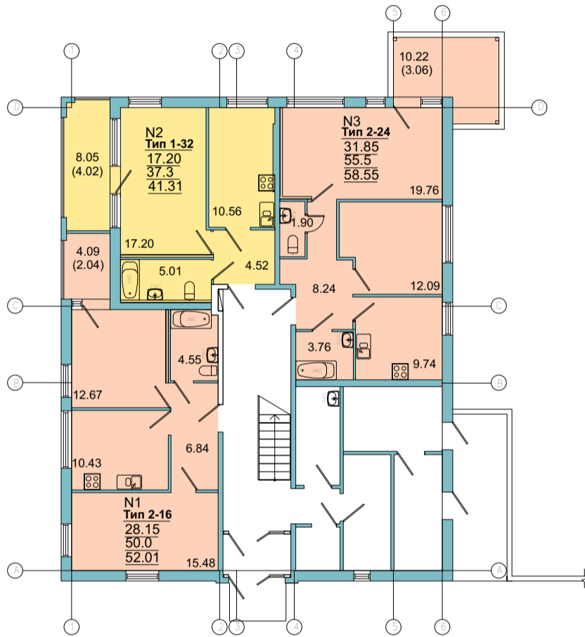
3 этаж (План на отм. +5,600)
