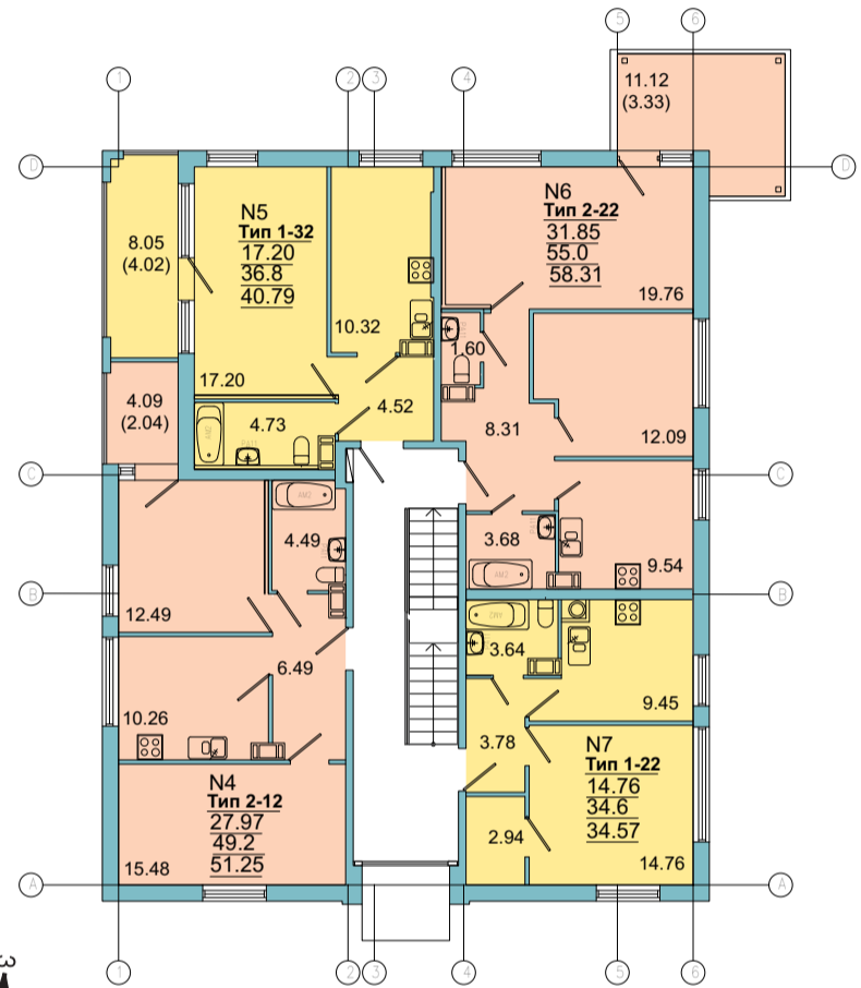
2 этаж (План на отм. +2,800)
